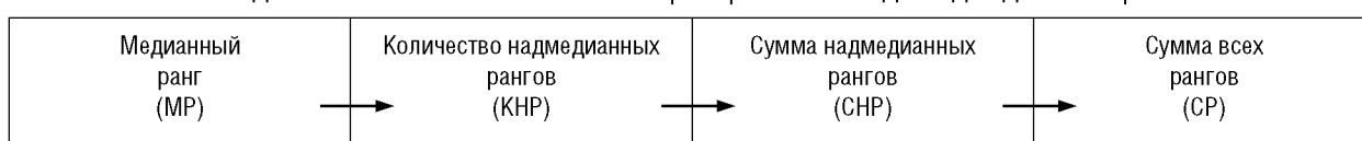
Последовательность использования критериев в методе надмедианных рангов
